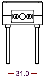
主视图 (1:2)
